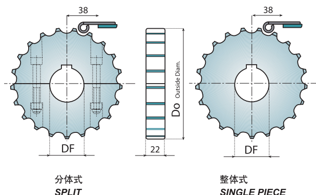
适用于 812-815MINI 链条 FOR CHAIN 812-815MINI
