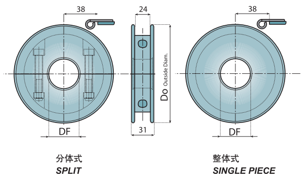
适用于 812-815MINI 链条 FOR CHAIN 812-815MINI
