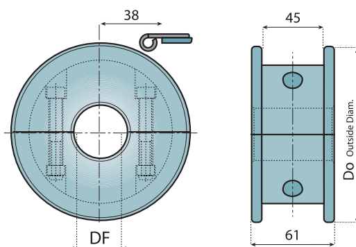
分体式从动轮 (机加工) SPLIT IDLER WHEEL ( MACHINED )
